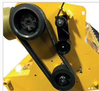
Napinacz automatyczny
