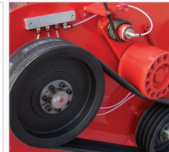
Smarowanie centralne
