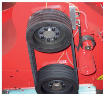
Automacyczny napinacz
