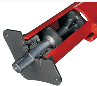
Wspornik rotora
